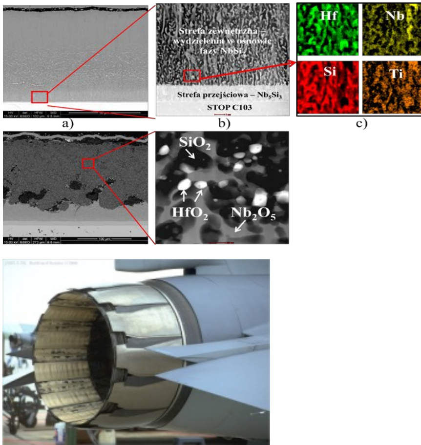
Technologia powłok żaroodpornych na stopach niobu
