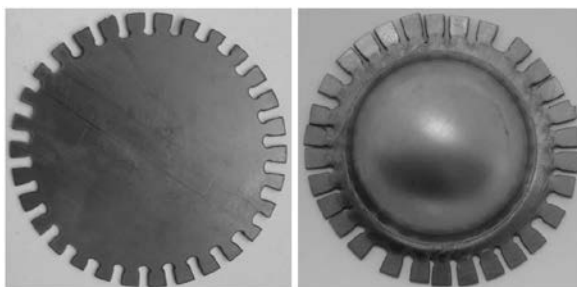
Wykrój oraz wytłoczka otrzymana z tytanu Ti-6Al-4V
