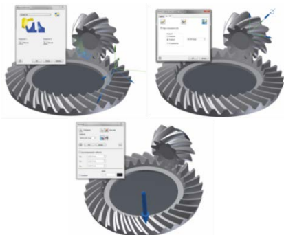
Sumaryczny ślad współpracy uzyskany na modelu bryłowym
