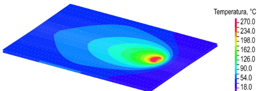
Rozkład temperatury w trakcie zgrzewania FSW
