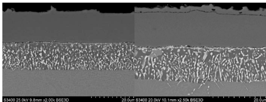
Mikrostruktura dyfuzyjnej warstwy aluminidkowej modyfikowanej cyrkonem wytworzona na podłożu stopu MAR M200+Hf (po lewej) oraz na łopatkę silnika lotniczego PZL-10 wykonanej ze stopu ZS6K
