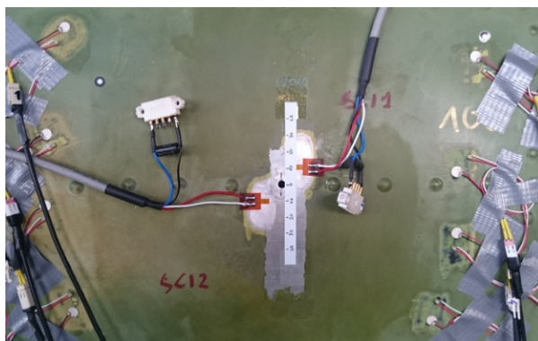
Przykład sieci PZT zainstalowanej na poszyciu belki ogonowej śmigłowca w celu monitorowania rozwoju pęknięcia zmęczeniowego
