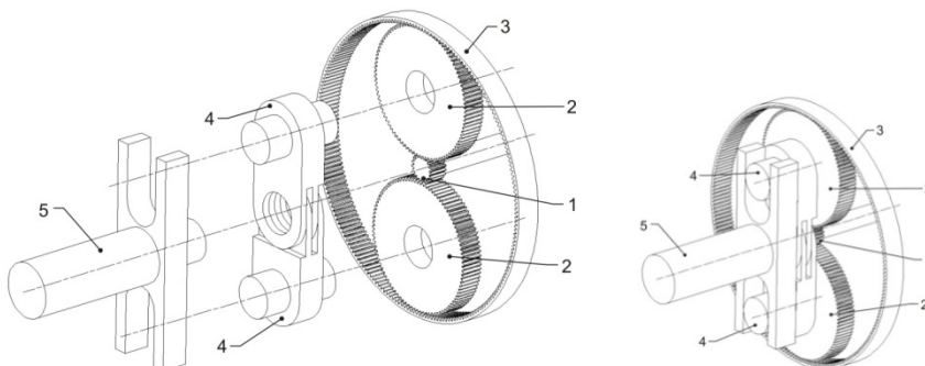
Przekładnia obiegowa z kasowaniem luzu międzyzębnego: a – złożona, b – częściowo zdemonstrowana; 1- zębniak, 2 – satelity, 3 – koło o uzębieniu wewnętrznym, 4 – dźwignie, 5 – wał wyjściowy z jarzmem
