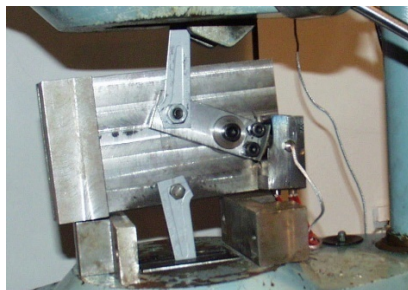
Stanowisko badawcze zamontowane na maszynie wytrzymałościowej
