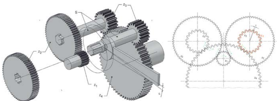
Schemat montażu; z_1, z_2, z_3, z_4 - koła zębate, S - wałki skrętne, \varepsilon - kąt napięcia wstępnego (odkształcenia)
