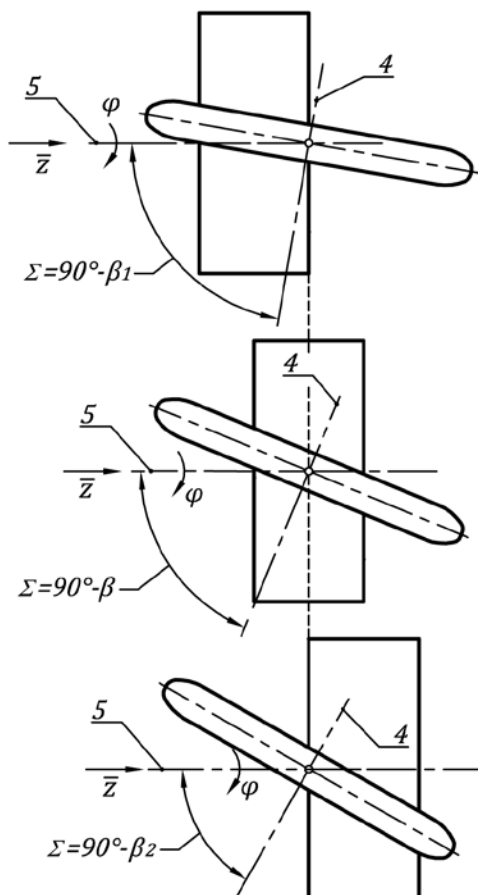
Schemat wprowadzania modyfikacji linii zębów wklęsłych w postaci fazowania
