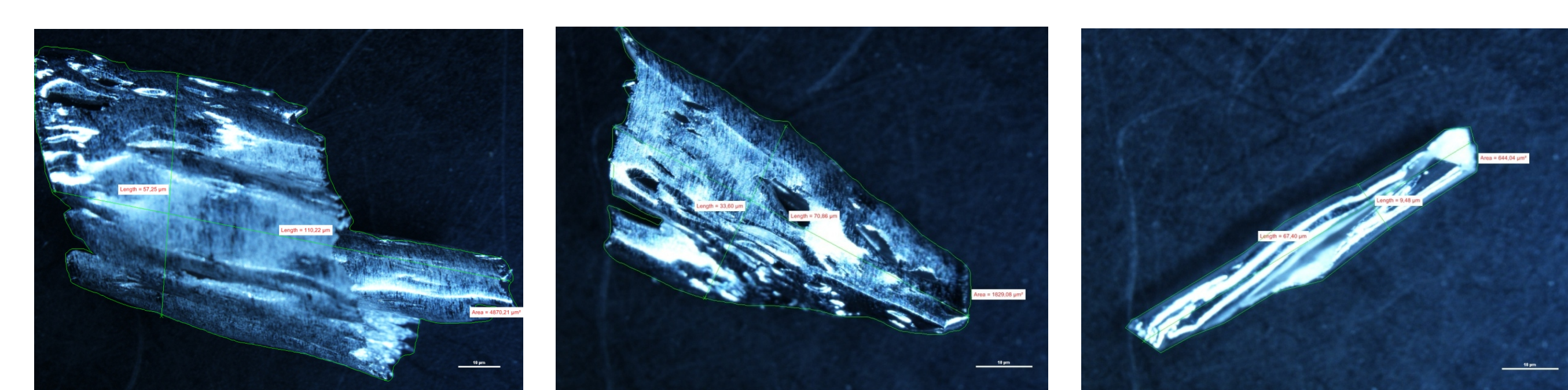
Rys. 4. Zarysy ścianek utwardzonych w przekrojach poprzecznych, długości ścianki 50mm; wartość wysięgu narzędzi: a) L=25mm; b) L=85mm Fig. 4. The outlines of constrained walls in cross-sections, the length of the wall 50mm; the value of outreach tools: a) L = 25mm, b) L = 85mm
