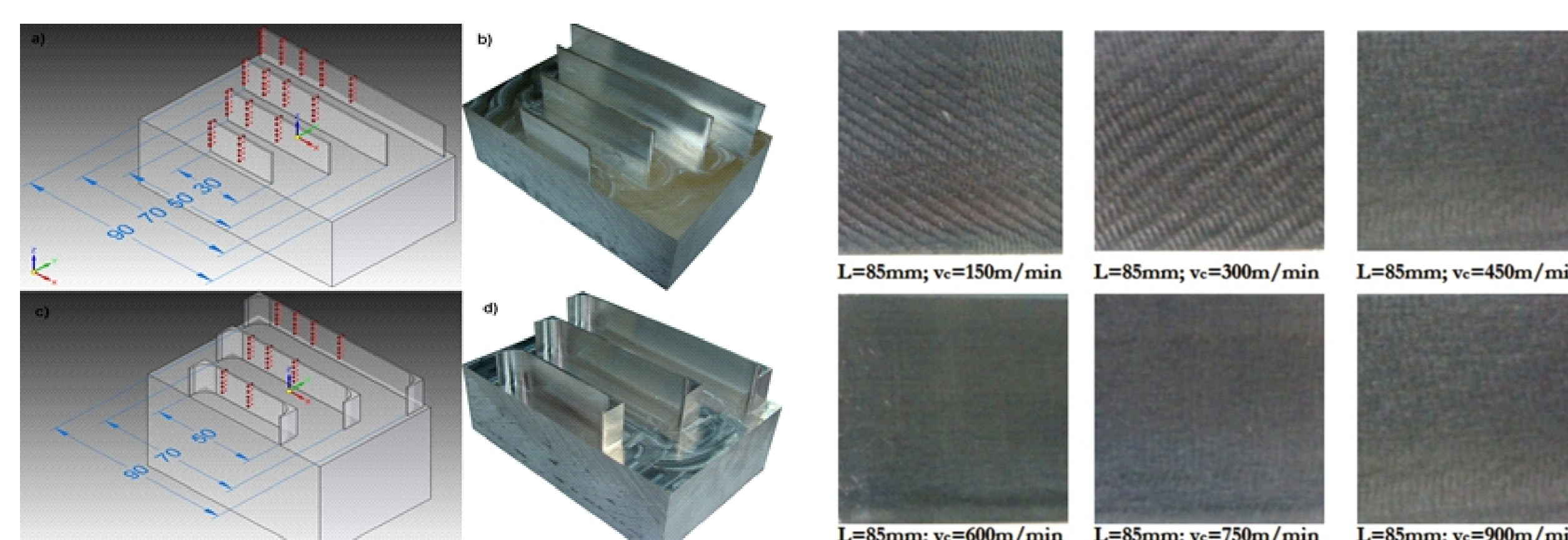
Rys. 2. Modele i widoki obrabianych próbek: a), b) próbki ze ściankami nieutwardzonymi; c), d) próbki ze ściankami utwardzonymi Fig. 2. Models and views machined samples: a), b) the sample with the unconstrained walls, c), d) the sample with the constrained walls
