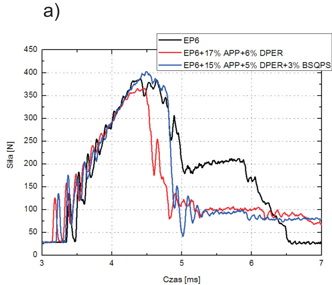
Rys. 3. Krzywe zmian siły w czasie rejestrowane podczas udarowego złamania próbek laminatów na osnowie EP6 oraz EP6 z dodatkiem antypirenów: a) szklanych, b) węglowych Fig. 3. Force curves as a function of time during impact fracture of laminates with matrix EP6 and EP6 containing flame retardant: a) glass, b) carbon
