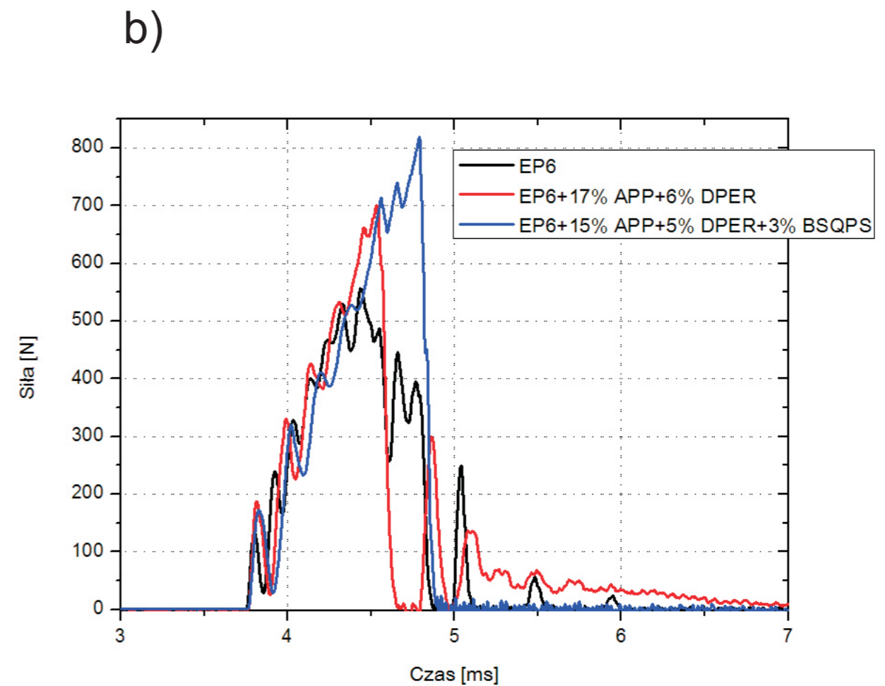
Rys. 3. Krzywe zmian siły w czasie rejestrowane podczas udarowego złamania próbek laminatów na osnowie EP6 oraz EP6 z dodatkiem antypirenów: a) szklanych, b) węglowych Fig. 3. Force curves as a function of time during impact fracture of laminates with matrix EP6 and EP6 containing flame retardant: a) glass, b) carbon
